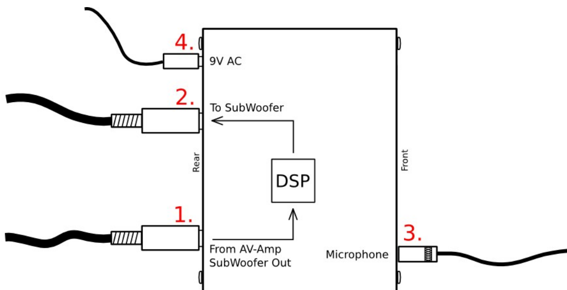
Afbeelding 3: Aansluiten van de ANTI-MODE 8033S
